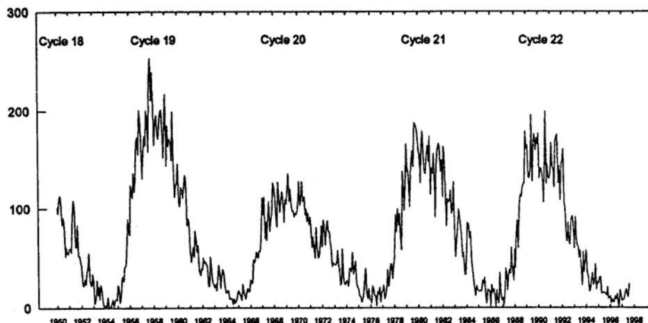
Figure 8-4. Les quatre derniers cycles de l'activité solaire
