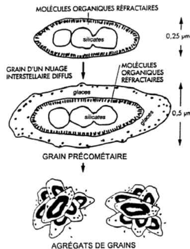
Figure 14-2. Du grain interstellaire à la comète
