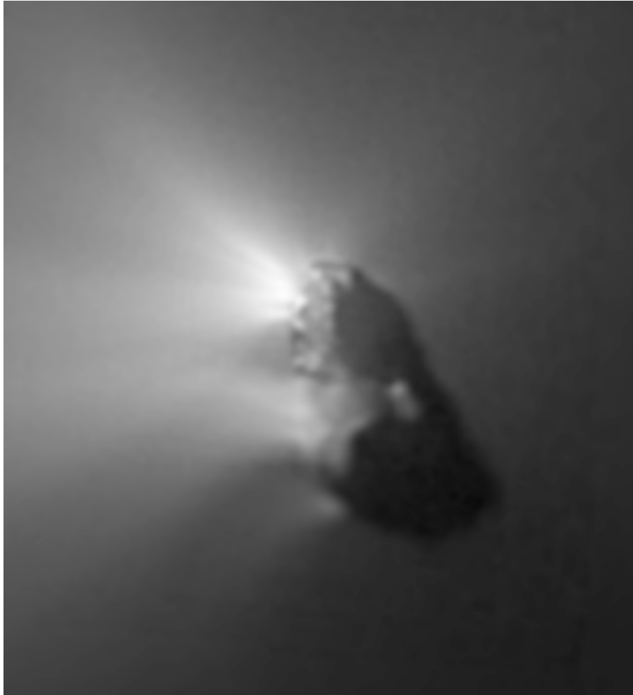
Figure 7-2. Première photographie du noyau d'une comète
