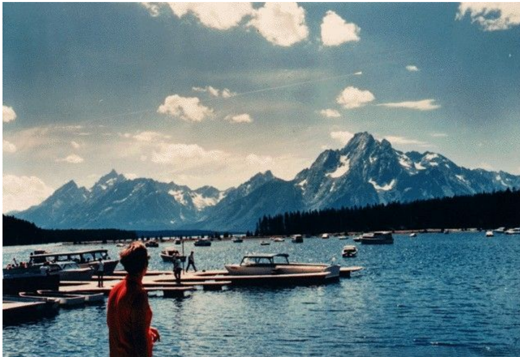
Figure 10-5. Le météore du Montana du 10 août 1972
