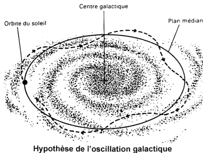
Figure 16-5. L'hypothèse de l'oscillation galactique
