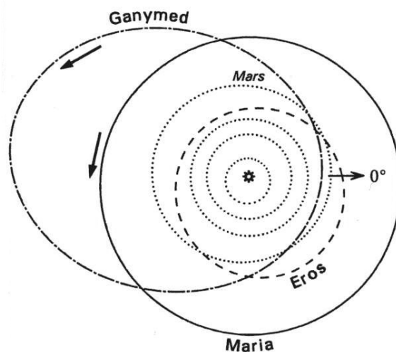
Figure 6-5. NEA, fragments d'un astéroïde brisé
