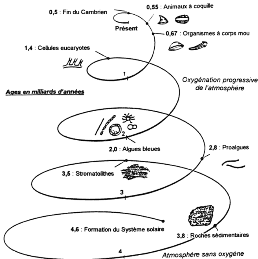
Figure 15-1. L'histoire biogéologique de la Terre
