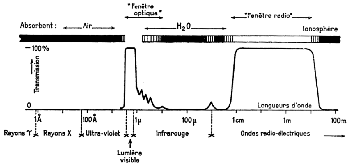
Figure 8-1. La gamme des rayonnements électromagnétiques
