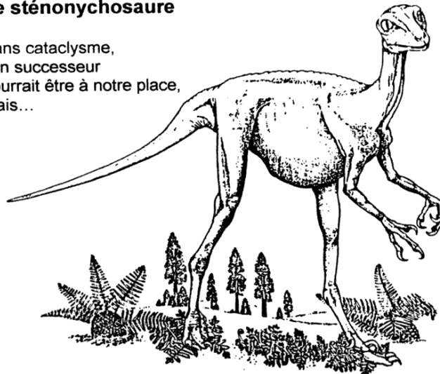
Figure 15-4. La fin du Crétacé et des Dinosaur
