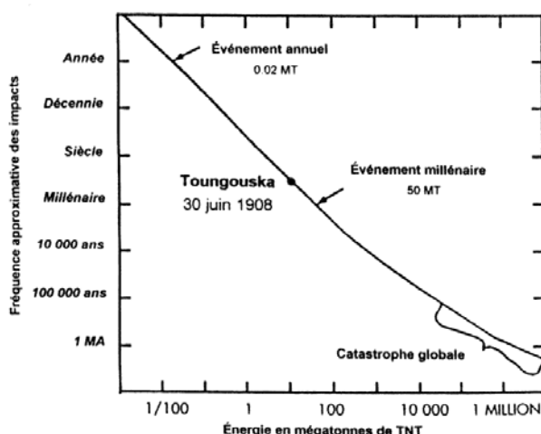
Figure 4-5. Le diagramme fréquence et énergie des impacts
