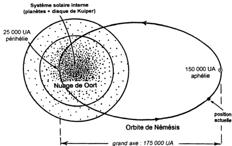
Figure 16-4. L'hypothèse Némésis, l'étoile sœur du Soleil
