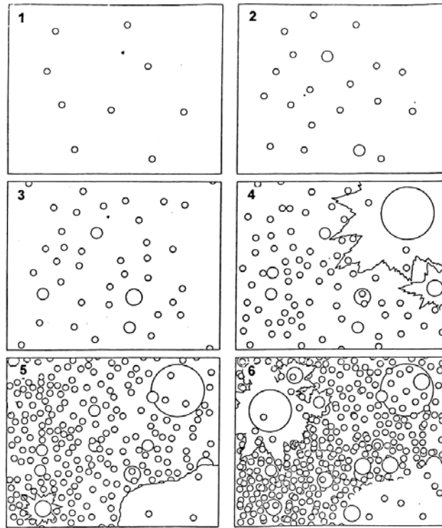
Figure 13-1. Le processus de cratérisation
