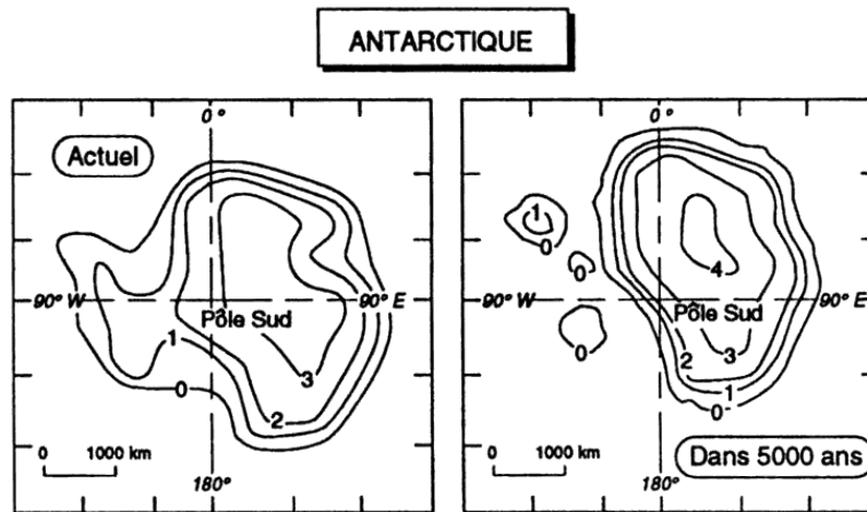
Figure 20-2. La déglaciation de l'Antarctique
