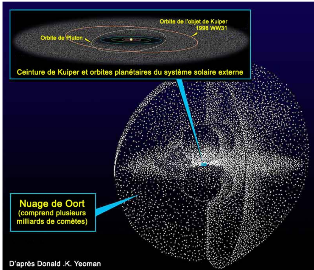
Figure 7-8. Le nuage de Oort
