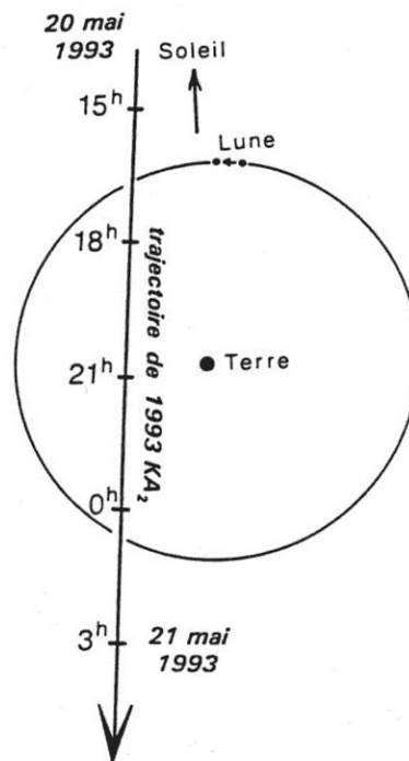
Figure 6-10. L'approche de 1993 KA 2 à la Terre le 20 mai 1993
