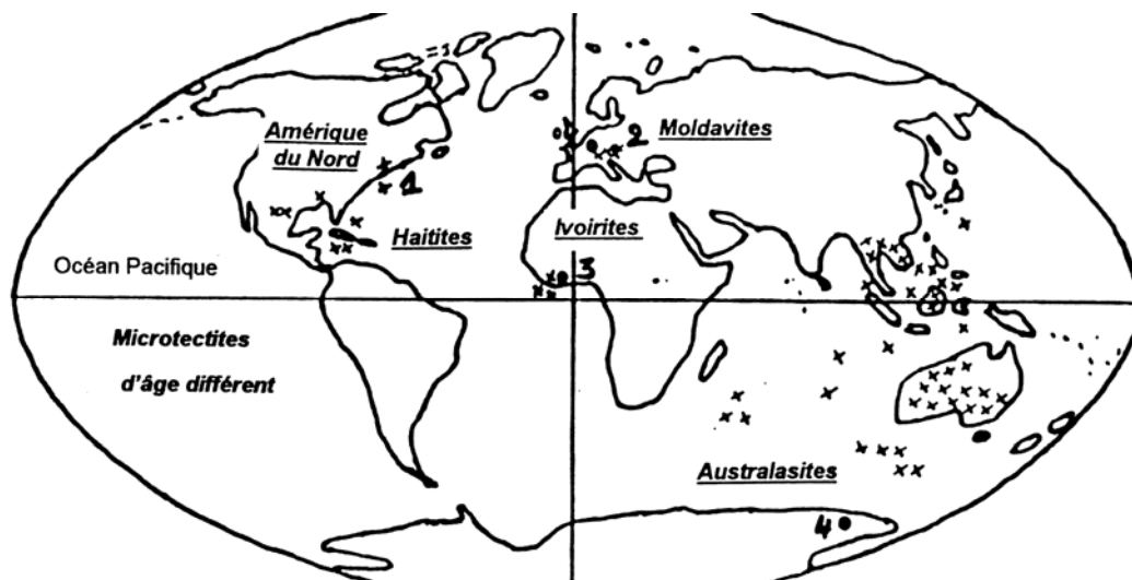
Figure 11-11. Les quatre grandes zones de tectites et les cratères parents
