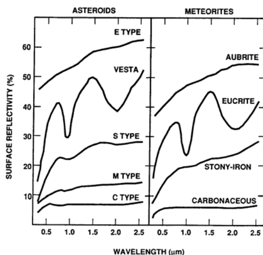
Figure 6-3. Comparaison entre les spectres des astéroïdes et des météorites
