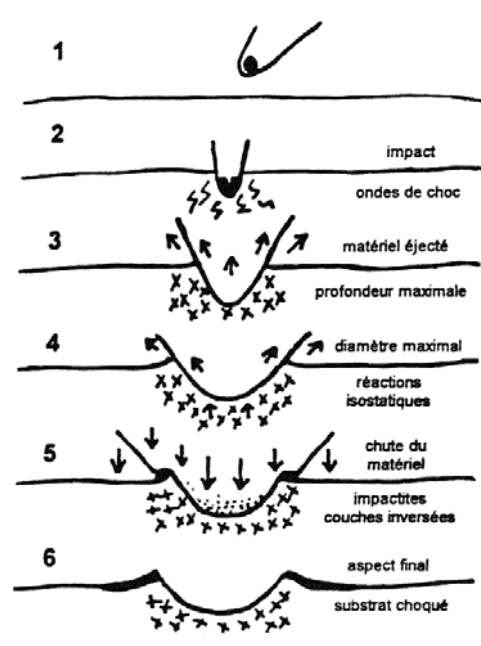
Figure 11-2. Formation d'un cratère météoritique
