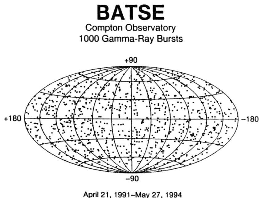
Figure 5-9. Les sursauts gamma : une origine extragalactique
