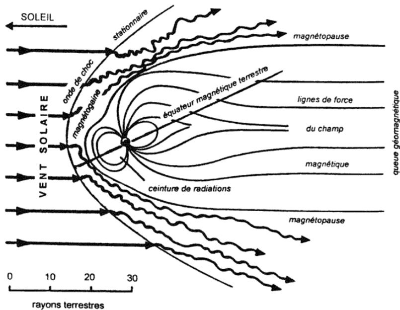
Figure 8-5. La magnétosphère terrestre
