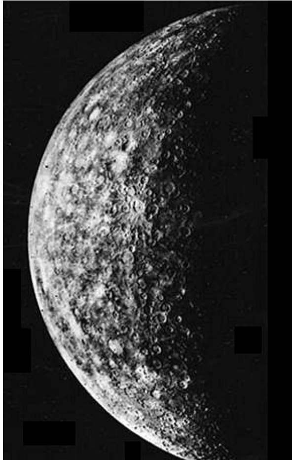
Figure 5-6. L'impactisme planétaire : la planète Mercure
