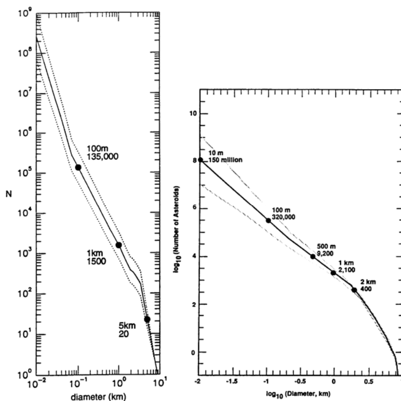
Figure 4-6. Le nombre estimé des NEA selon leur diamètre
