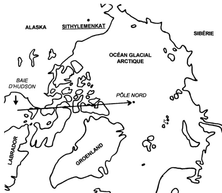
Figure 19-1. Le dernier déplacement du pôle géographique (hypothétique)
