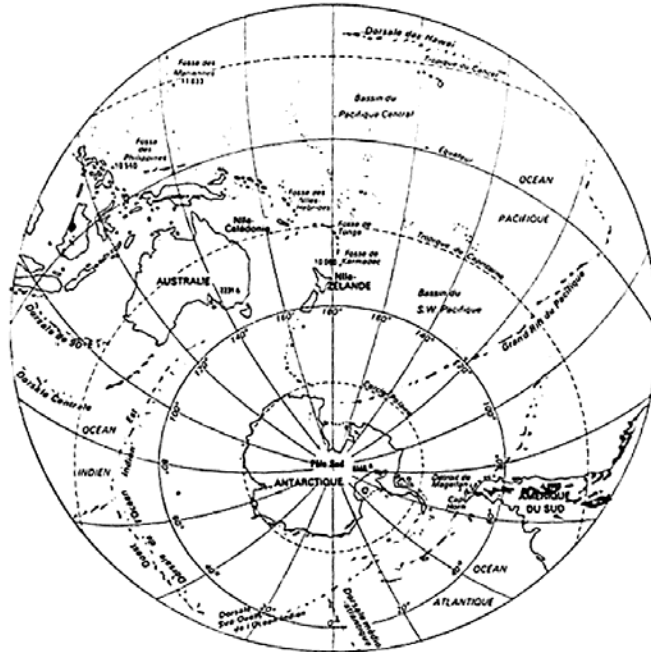
Figure 13-7. L'Antarctique : un continent excentré
