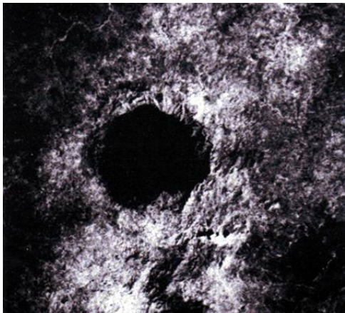
Figure 11-10. Bosumtwi : le cratère parent des ivoirites Ce cratère ghanéen de 10 km de diamètre date de 1 MA et a été créé par l'impact d'un astéroïde de 500 mètres de diamètre. A noter que cette structure est associée aux ivoirites, l'une des familles de tectites. Il est associé également à une inversion géomagnétique, bien qu'il ne soit pas certain que les deux événements soient liés génétiquement. (Document NASA).
