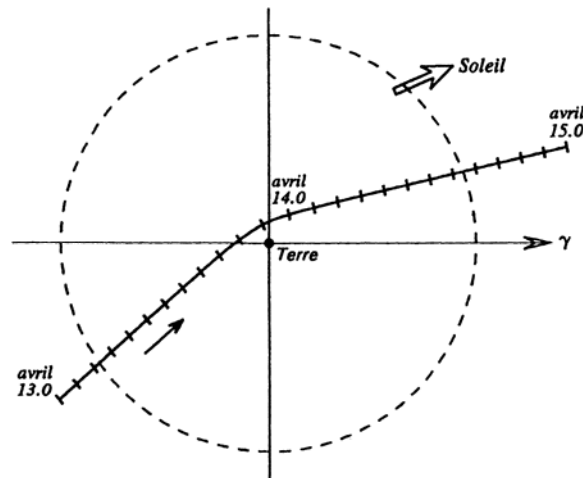
Figure 6-13. L'approche d'Apophis en avril 2029
