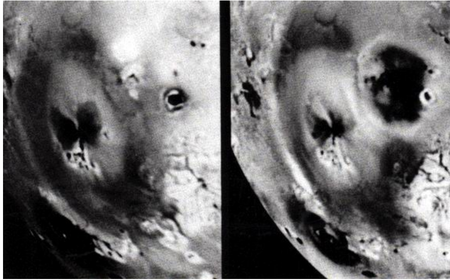
Figure 5-17. Volcanisme dans le Système solaire
