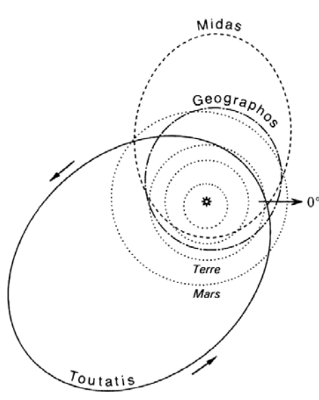
Figure 6-2. Les sous-types de NEA de type Apollo
