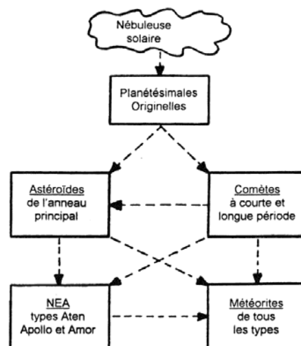
Figure 5-3. Origine et évolution des petits corps du Système solaire
