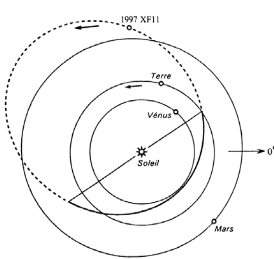
Figure 17-7. L'orbite de 1997 XF 11 , "l'astéroïde de l'Apocalypse"
