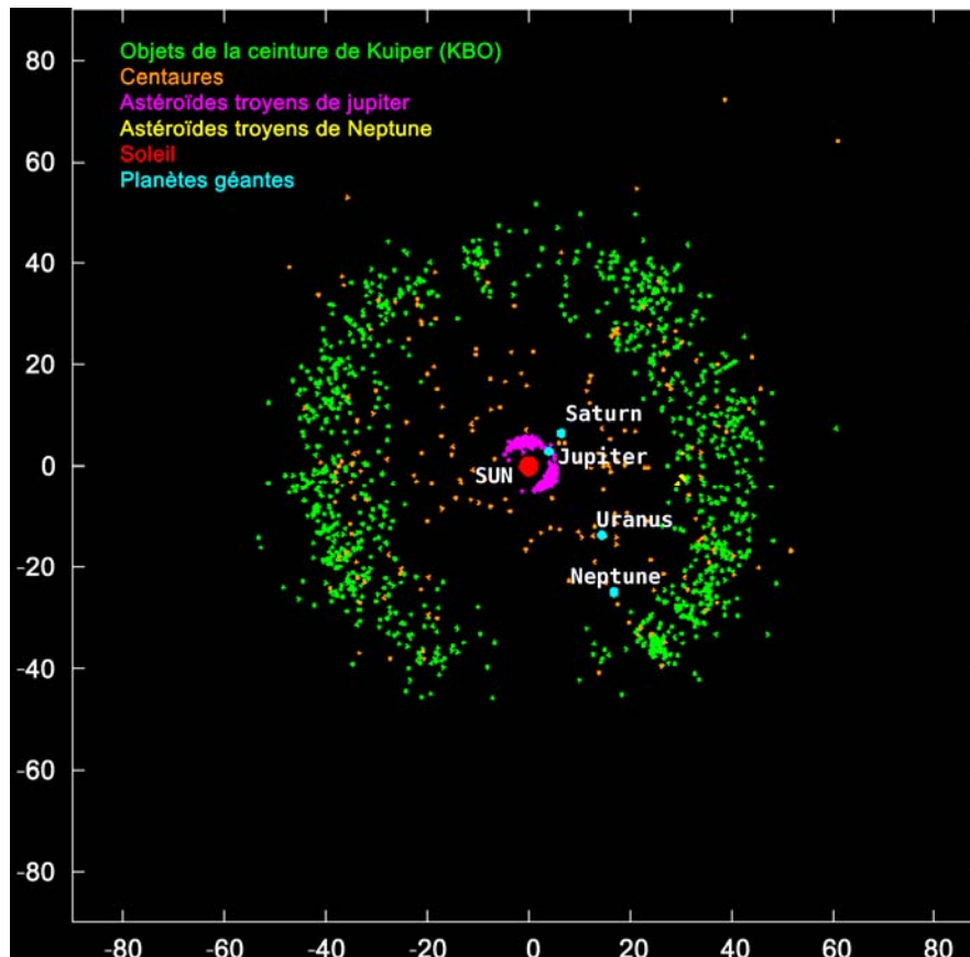
Figure 7-10. La ceinture de Kuiper : une nouvelle population d'objets
