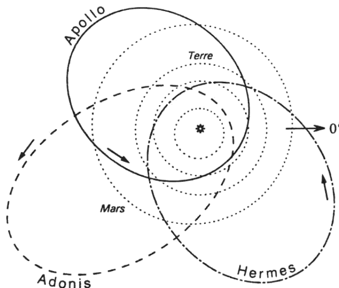
Figure 4-3. Les orbites d'Apollo, Adonis et Hermès
