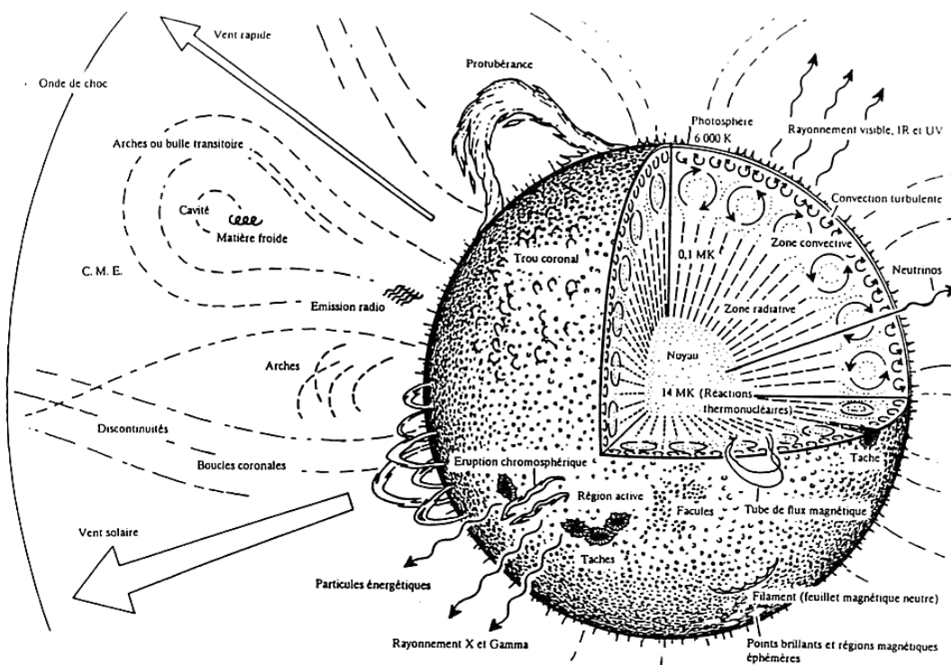
Figure 8-2. La structure du Soleil et ses rayonnements
