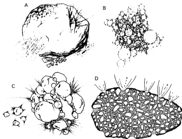
Figure 7-1. Quatre modèles de structure de noyaux cométaires
