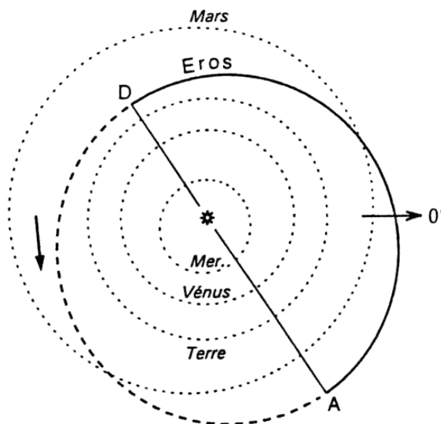
Figure 4-2. Eros, l'astéroïde qui a tout changé
