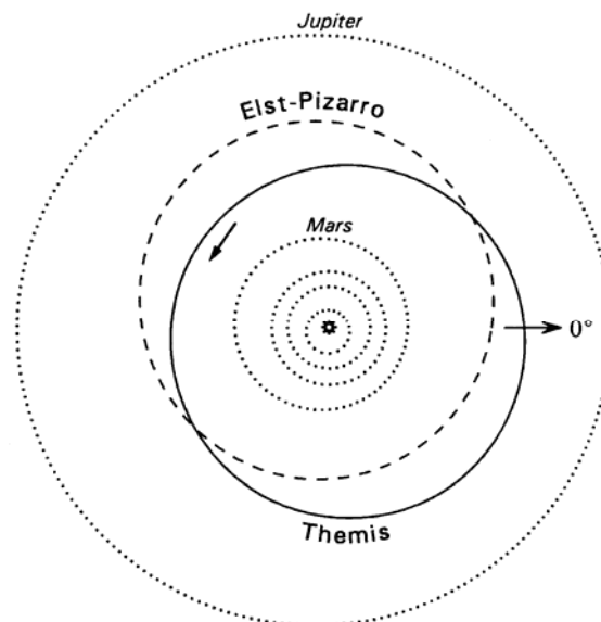
Figure 6-6. Astéroïde cométaire, membre d'une famille d'astéroïdes
