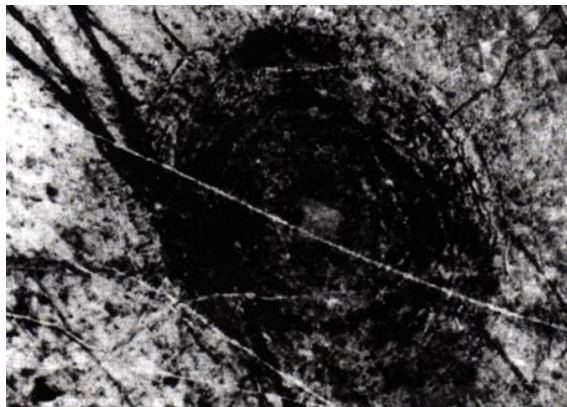
Figure 5-7. L'impactisme planétaire : l'exemple d'Europa
