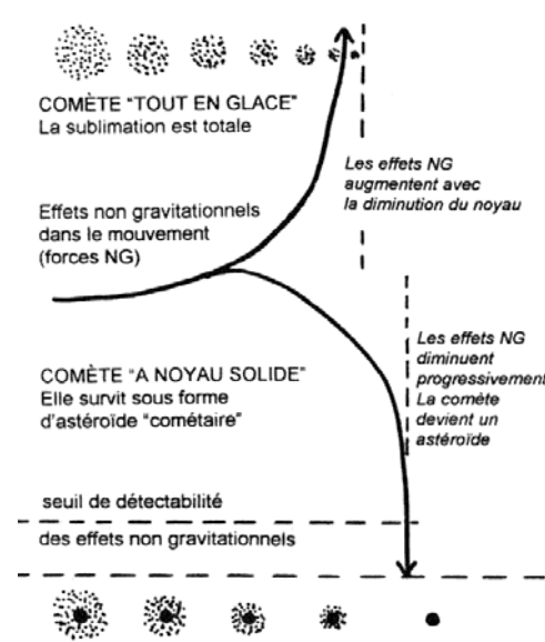
Figure 7-4. L'évolution d'un noyau cométaire "tout en glace" et "à noyau solide"
