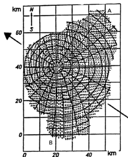
Figure 9-3. La région sinistrée de la Tougouska
