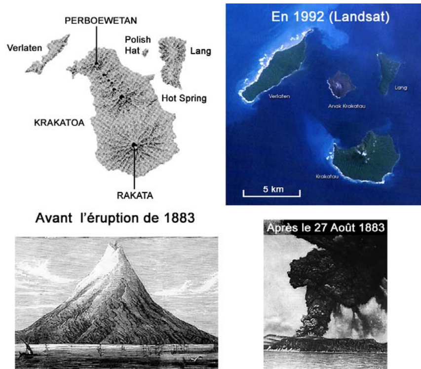
Figure 6-14. Eruptions volcaniques : l'explosion du Krakatoa en 1883
