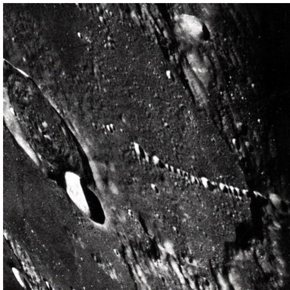
Figure 5-16. La chaîne de craterlets Catena Davy sur la Lune
