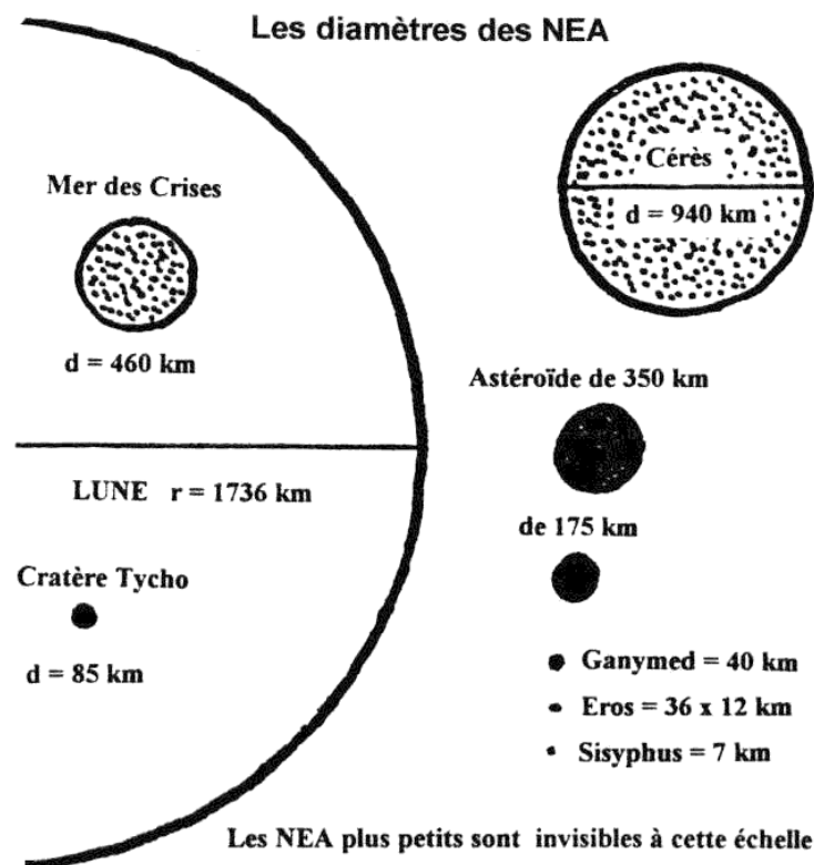
Figure 6-8. Diamètres comparés de la Lune, Cérès et de NEA
