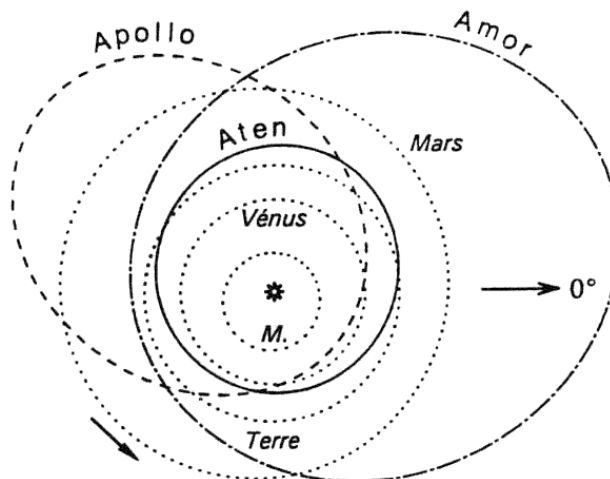
Figure 6-1. Les trois types de NEA
