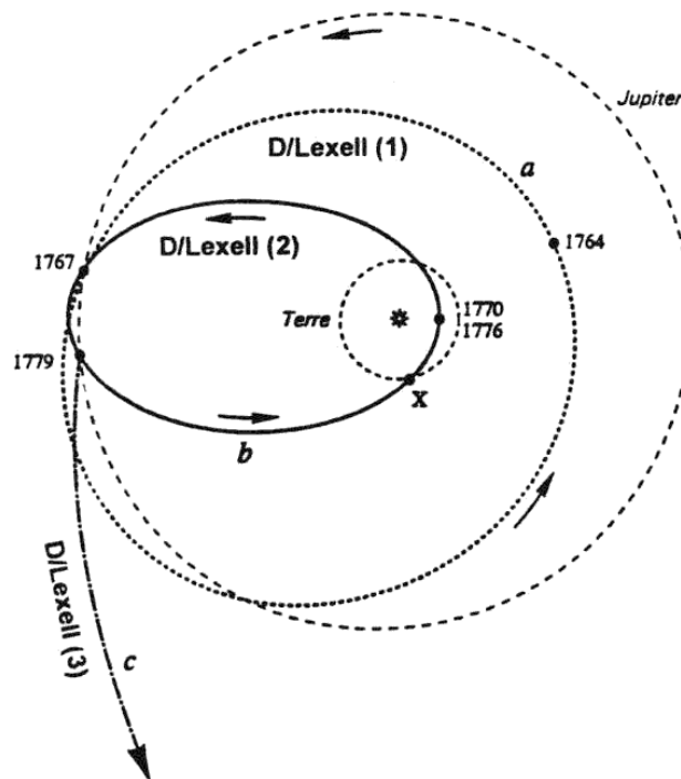
Figure 7-6. L'orbite de la comète D/Lexell entre 1760 et 1780
