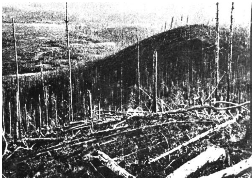
Figure 9-4. L'étude photographique de la région dévastée
