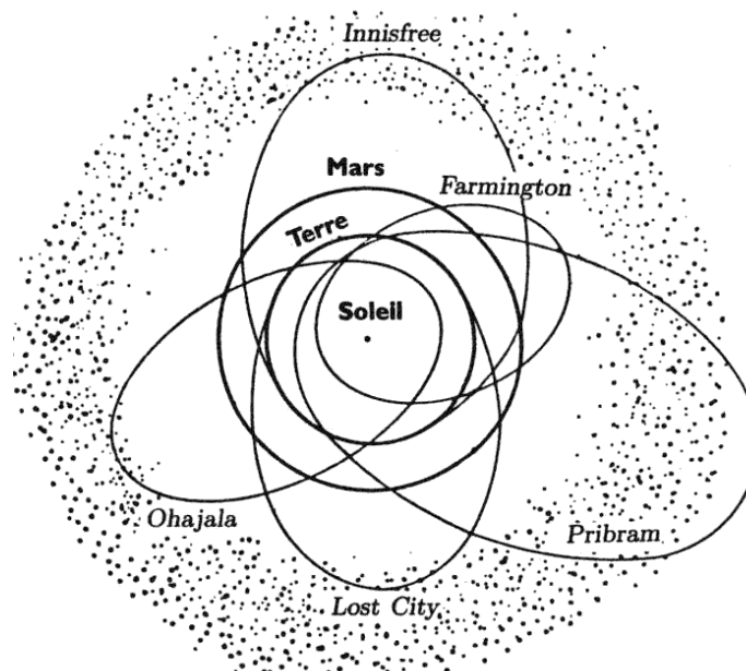
Figure 10-9. Orbites préatmosphériques de cinq météorites
