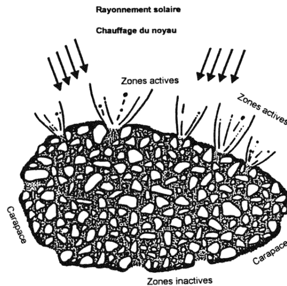
Figure 7-16. Structure d'un noyau cométaire mixte
