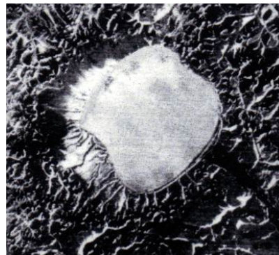
Figure 11-8. Un grand astroblème récent en Sibérie : Elgygytgyn
