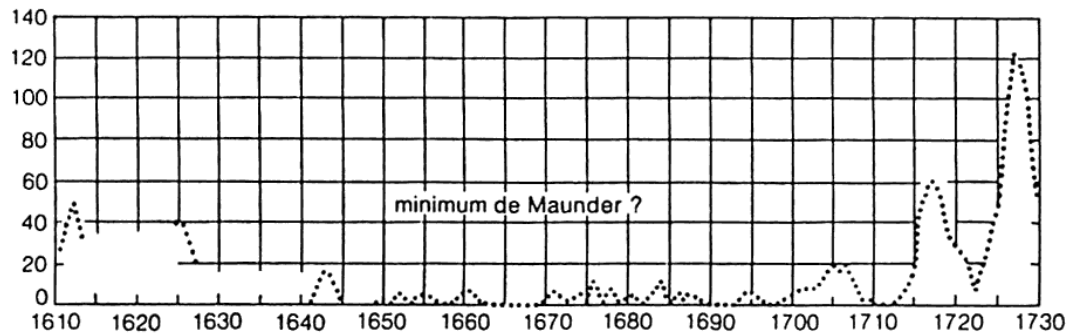
Figure 20-6. Les bas et les hauts de l'activité solaire
