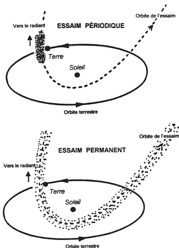
Figure 10-7. Essaims de météores périodiques et permanents
