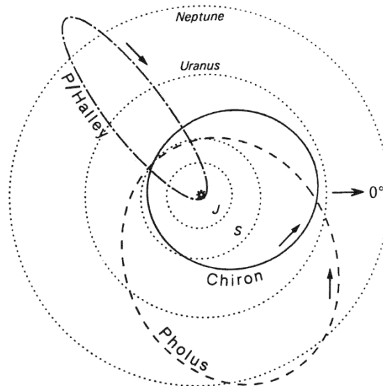
Figure 7-11. La région des centaures et P/Halley
