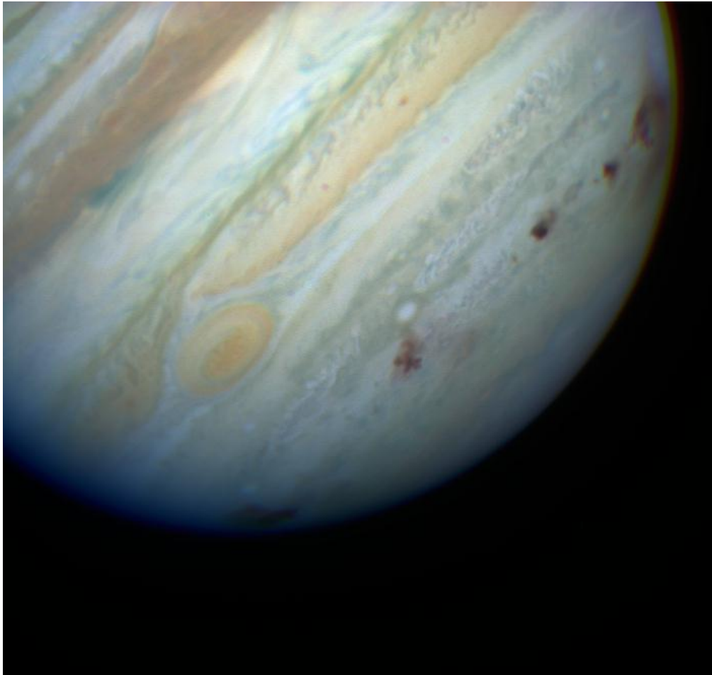
Figure 5-14. Traces d'impact de SL9 sur Jupiter
