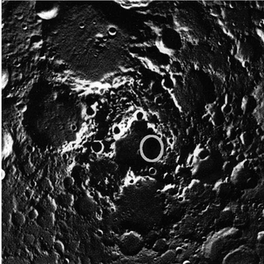
Figure 5-5. L'impactisme lunaire : astéroïdes et comètes
