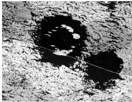
Figure 11-5. Les Clearwater Lakes : deux astroblèmes jumeaux
