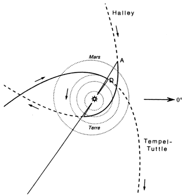
Figure 7-5. Les orbites de P/Halley et de P/Tempel-Tuttle
