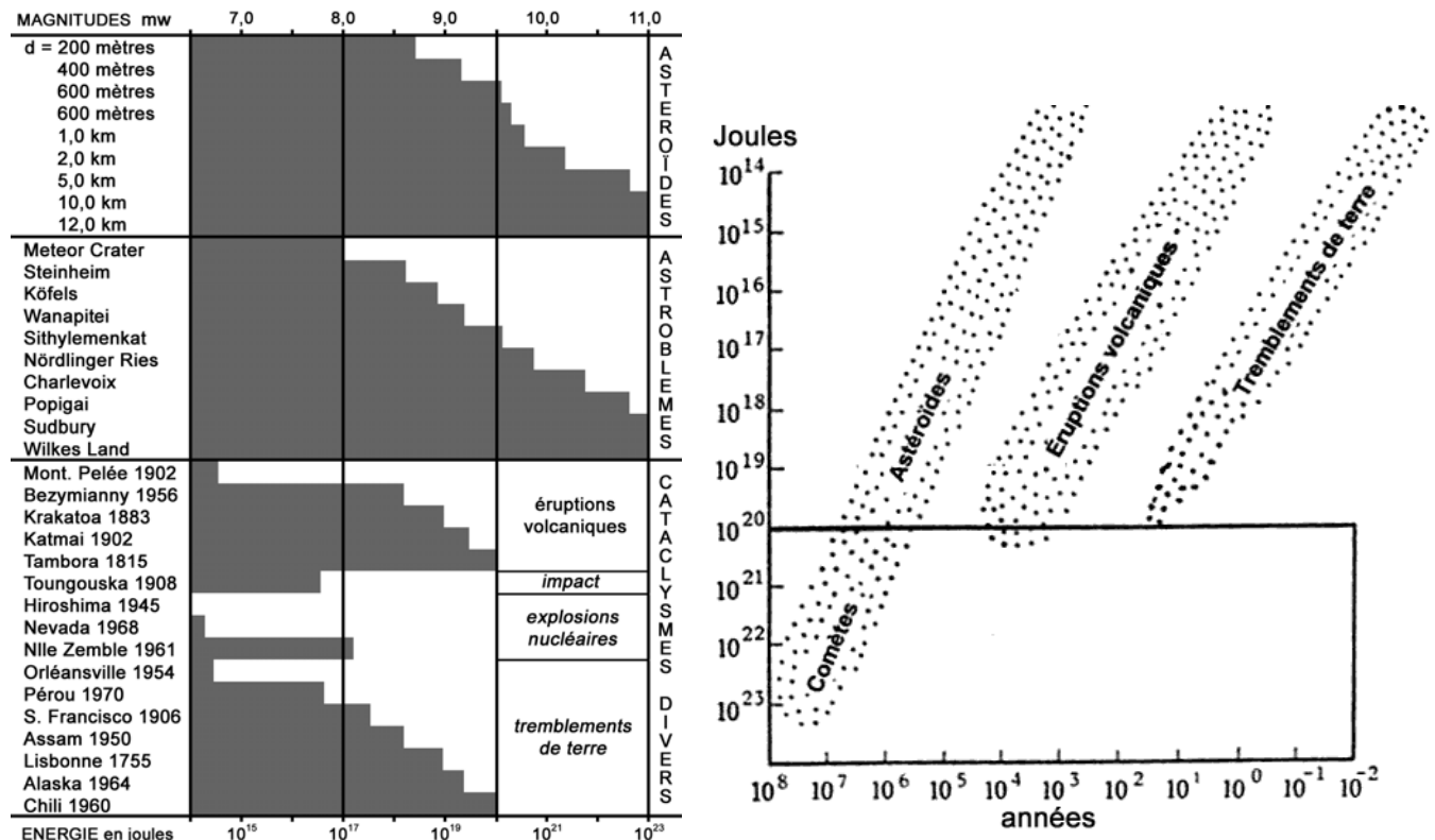
Figure 6-15. Énergie comparée et fréquence des impacts et des cataclysmes terrestres
