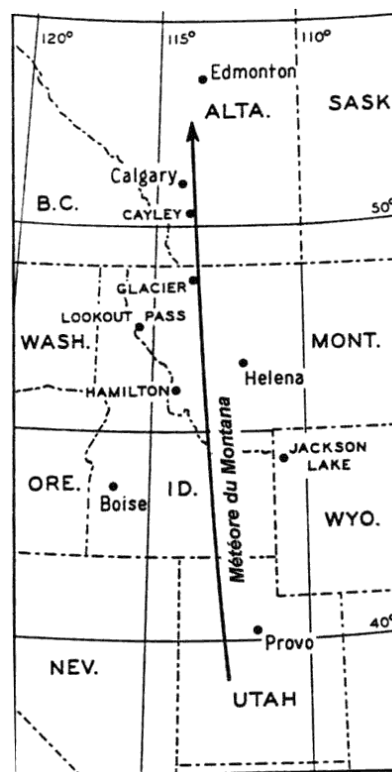
Figure 10-4. Trajectoire du météore du Montana du 10 août 1972
