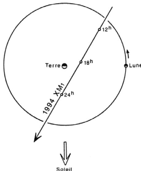
Figure 6-11. L'approche de 1994 XM 1 à la Terre le 9 décembre 1994
