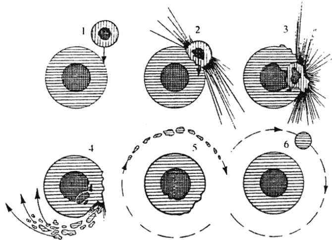
Figure 13-2. Mécanisme de formation de la Lune
