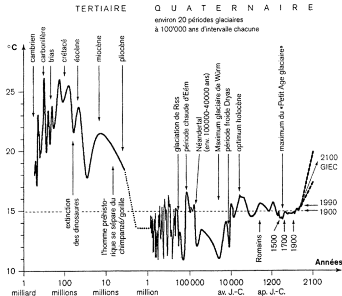
Évolution de la température terrestre depuis 600 millions d'années
