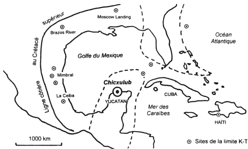
Figure 12-6. Chicxulub : la région de l'impact
