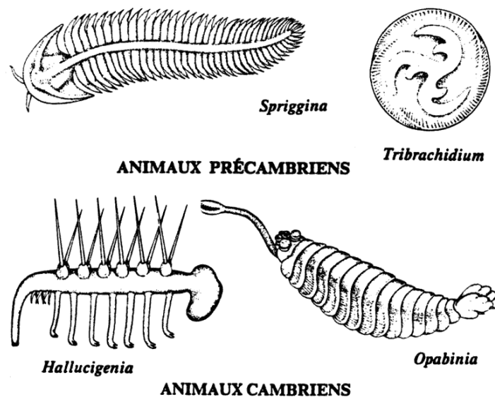
Figure 15-2. L'explosion de la vie : le Précambrien et le Cambrien
