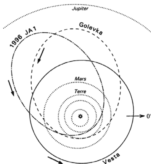
Figure 6-4. NEA, éclats d'un astéroïde
