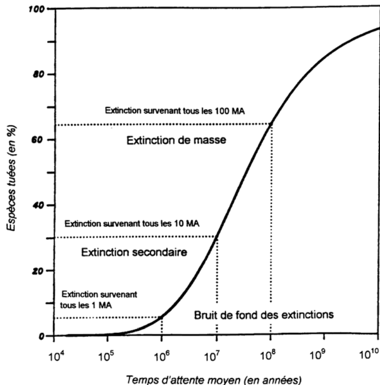
Figure 15-3. Courbe des espèces tuées
