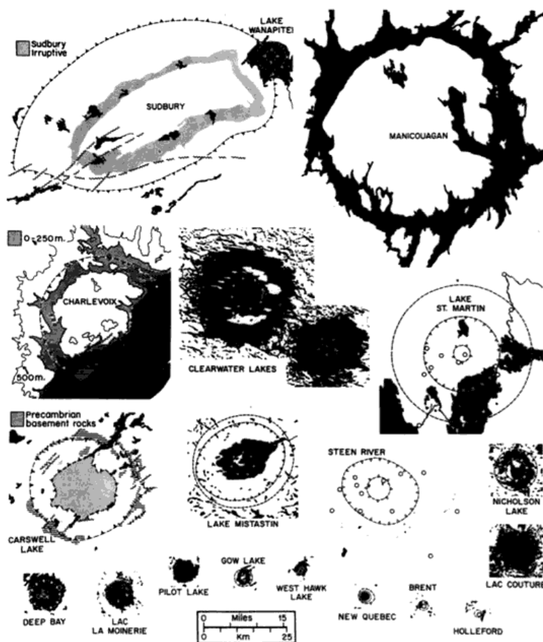
Figure 11-3. Les astroblèmes canadiens
