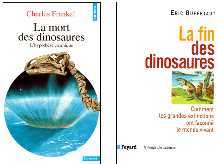
Figure 12-8. Le cataclysme, élément majeur de l'histoire de la vie
