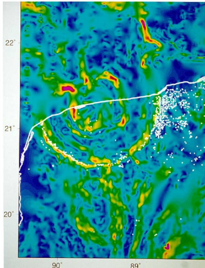
Figure 12-4. Chicxulub : les traces gravimétriques de l'impact
