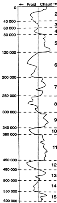
Figure 13-4. La théorie astronomique des climats et les périodes glaciaires
