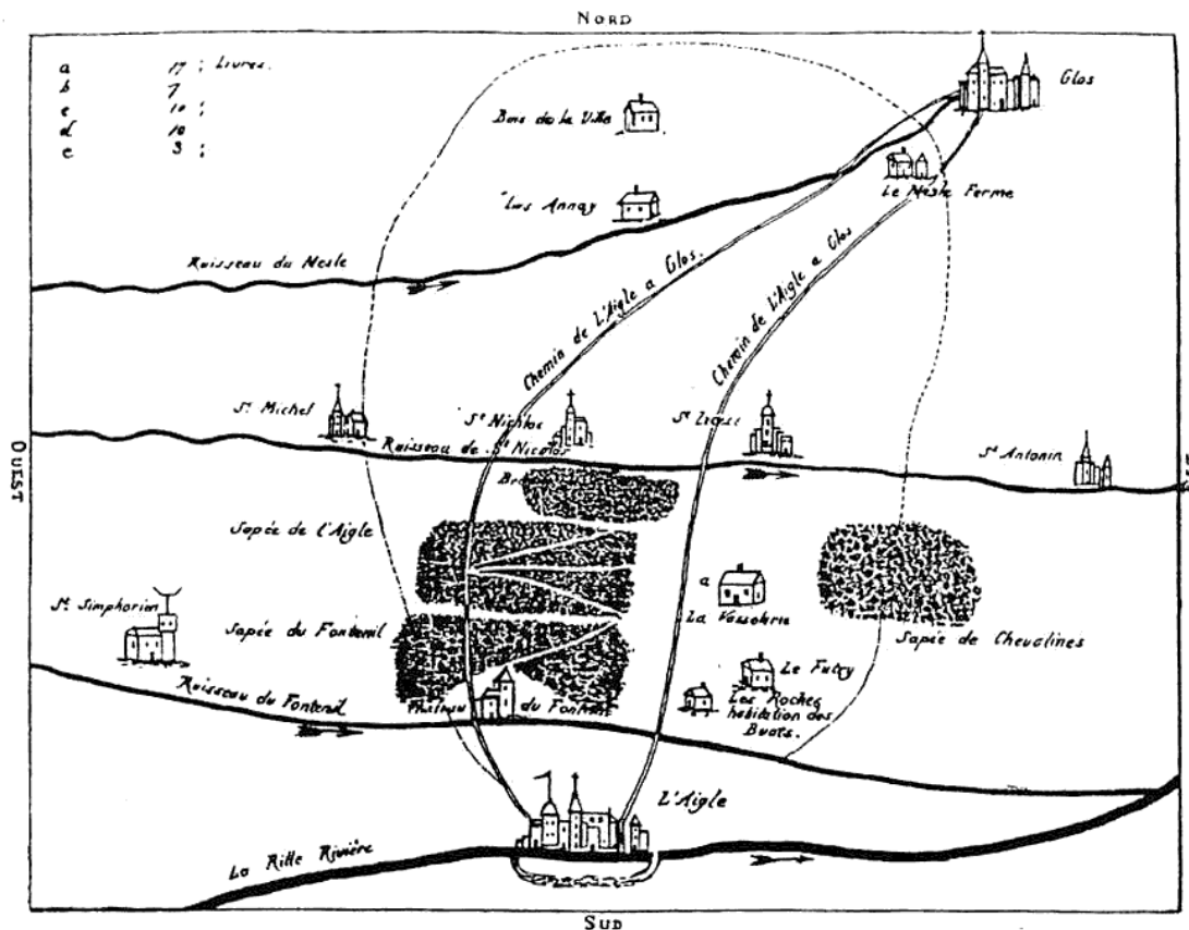
Figure 3-5. Carte de la région de L'Aigle et zone de distribution des météorites
