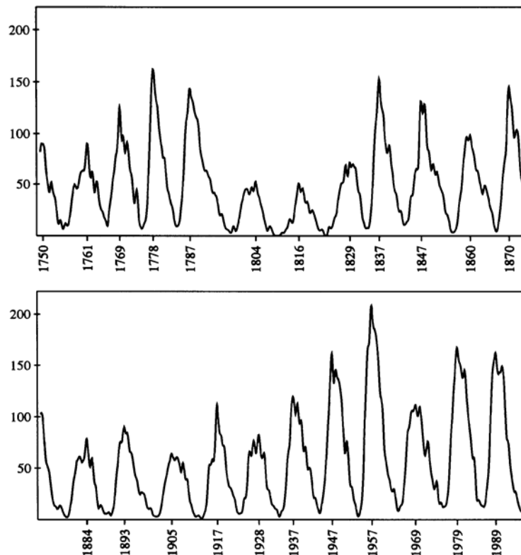
Figure 8-3. Le Soleil et ses cycles d'activité
