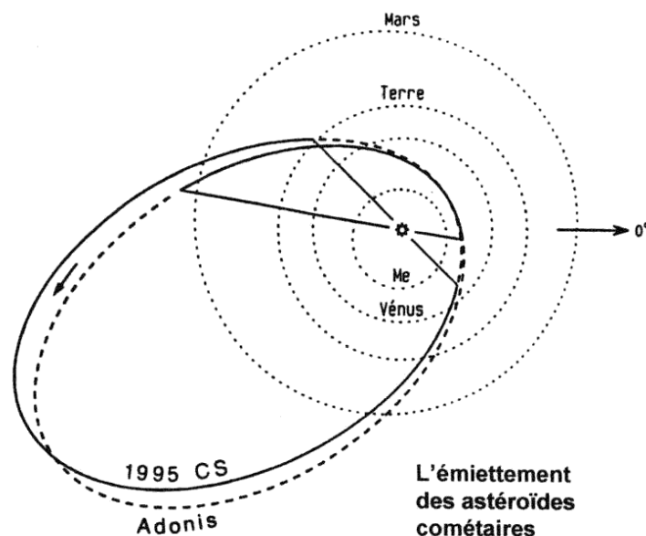
Figure 6-7. L'émiettement des astéroïdes cométaires
