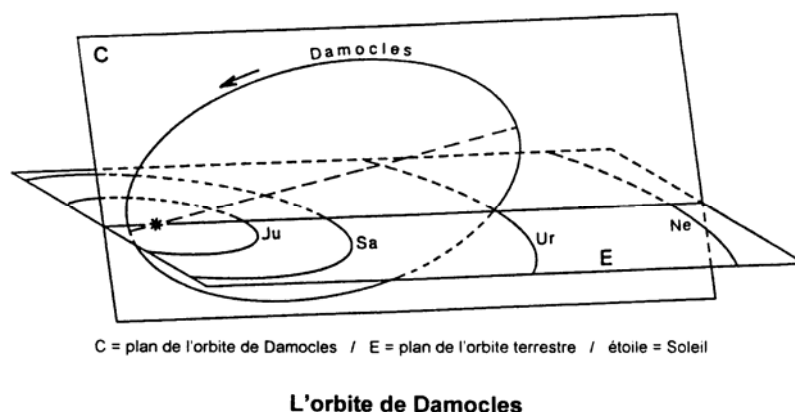
Figure 7-12. Damocles : du nuage de Oort à la banlieue solaire
