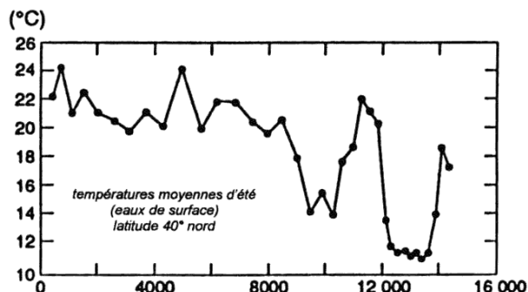
Figure 19-2. Les variations de température depuis 15 000 ans
