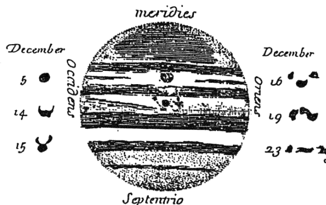
Figure 5-15. Un impact de comète sur Jupiter en 1690 ?
