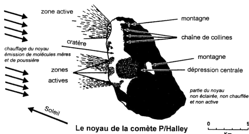
Figure 7-3. Le noyau de la comète P/Halley
