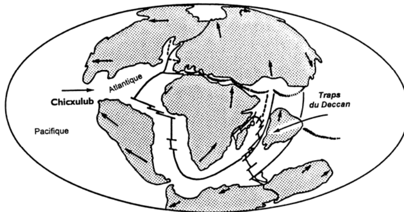
Figure 12-2. La géographie terrestre à la fin du Crétacé
