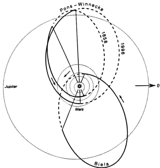
Figure 7-7. Les orbites de D/Biela et P/Pons-Winnecke
