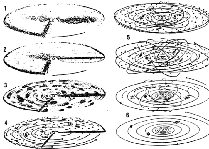
Figure 5-2. La formation du Système solaire
