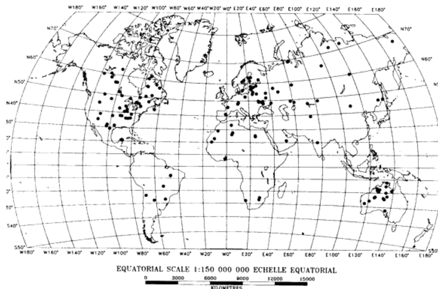
Figure 11-6. Les astroblèmes terrestres recensés
