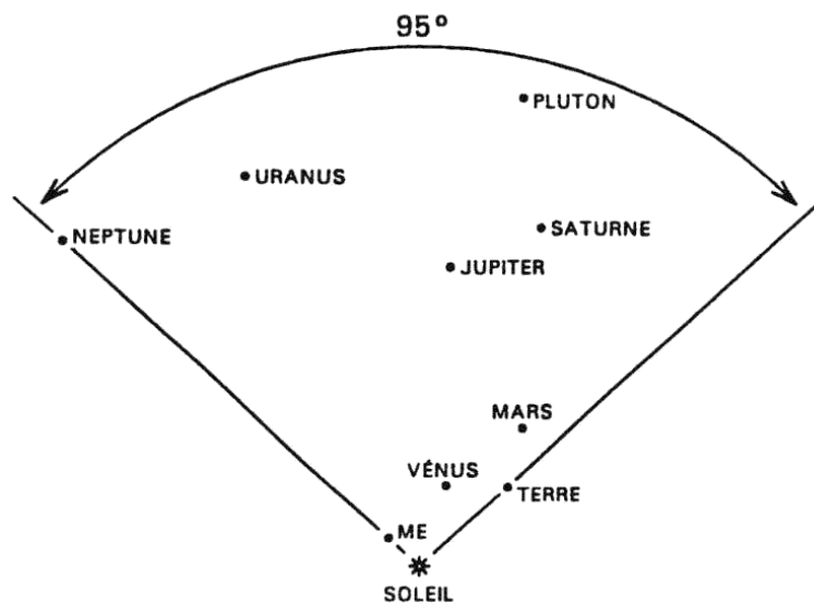
Groupeement des planètes du 10 mars 1982
