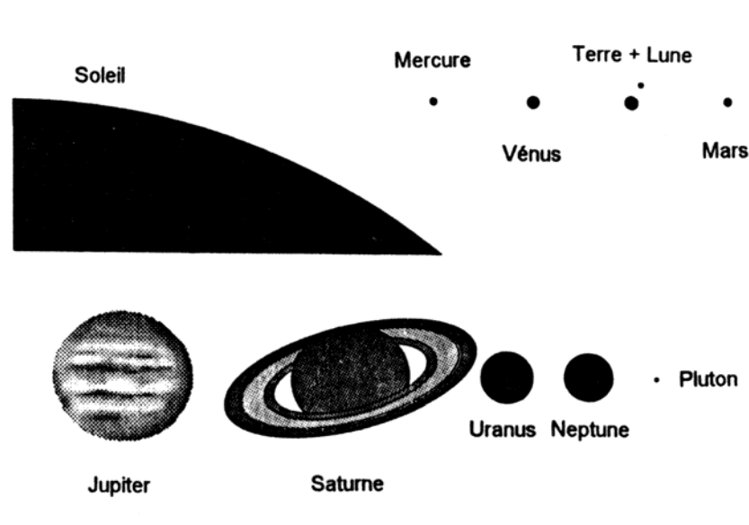
Figure 6-9. Les NEA : de la poussière cosmique à l'échelle astronomique
