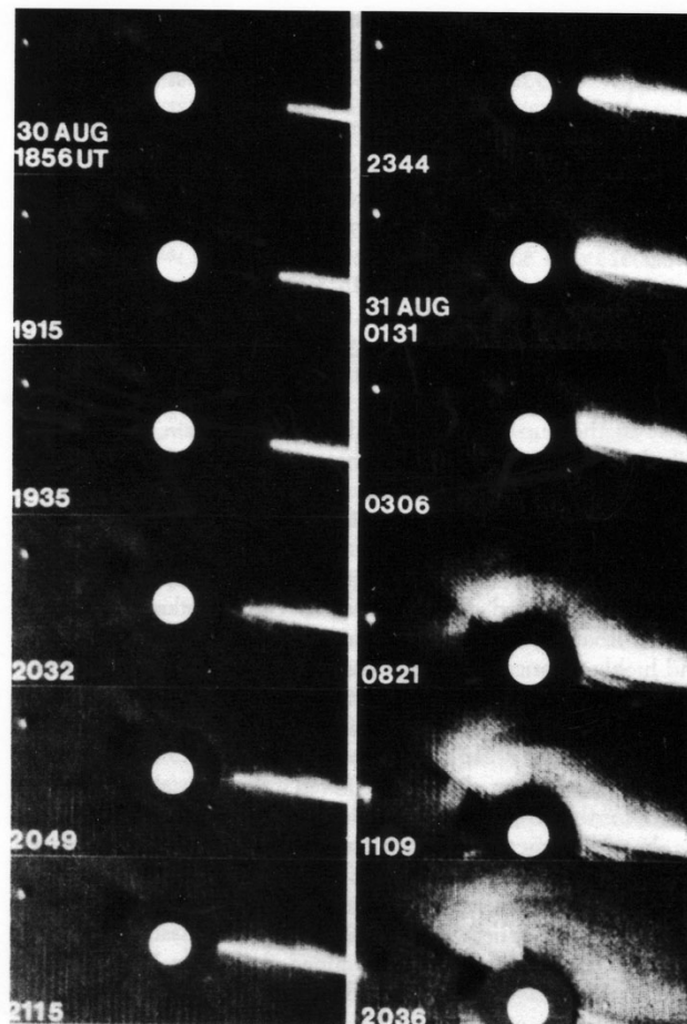
Figure 7-14. La mort d'une comète : collision avec le Soleil
