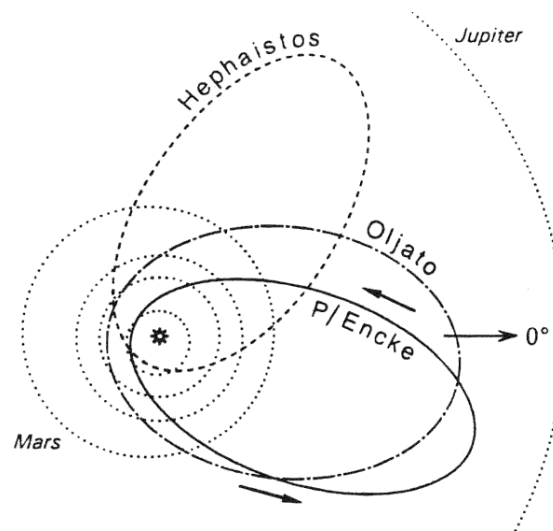
Figure 7-15. Les orbites de Hephaistos, Oljato et P/Encke
