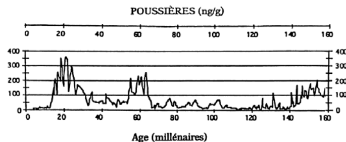
Figure 13-5. La poussière piégée dans les glaces
