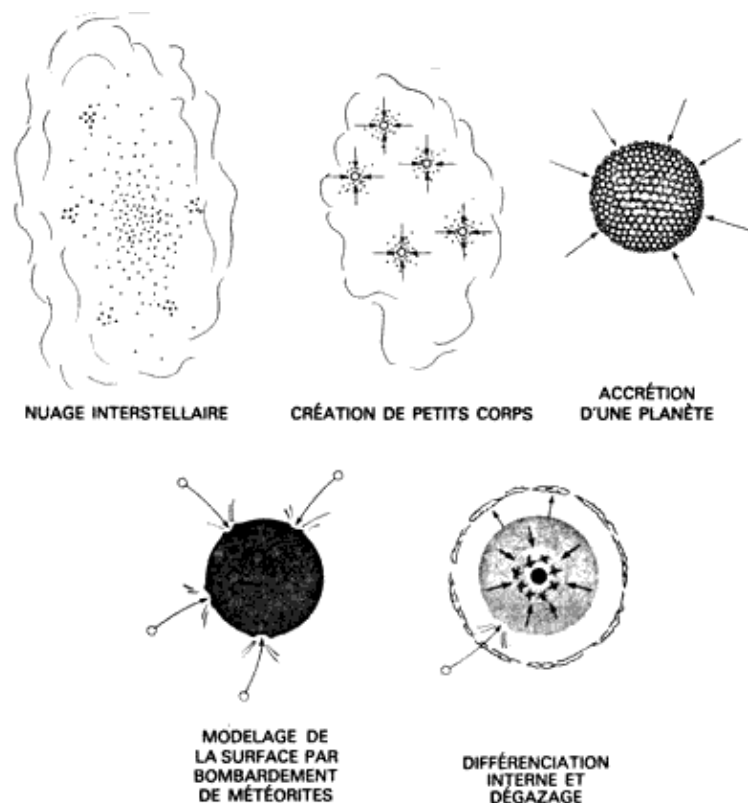
Figure 5-4. La formation des planètes
