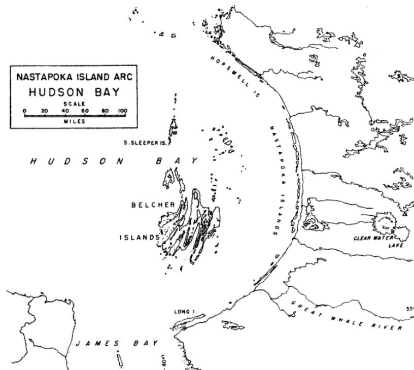
Figure 11-9. La possibilité d'astroblèmes géants
