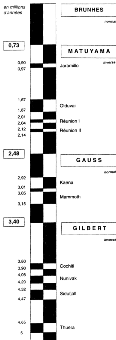
Figure 13-6. Les variations du champ géomagnétique depuis 5 millions d'années
