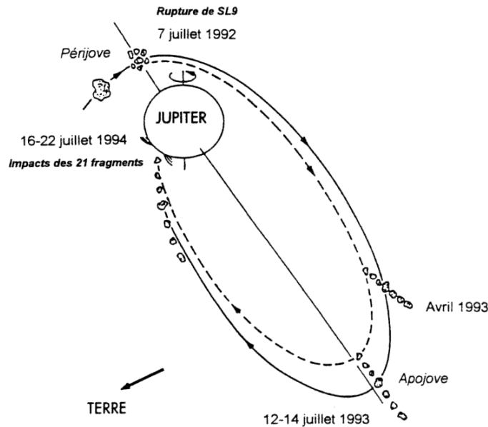
Figure 5-13. La dernière orbite de SL9 entre juillet 1992 et juillet 1994
